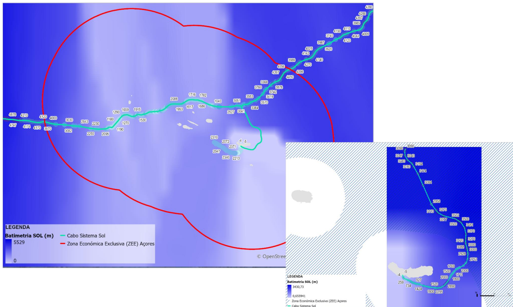
Figura 7.2 - Profundidade (batimetria) para instalação do cabo SOL e respetivas batimetrias na ZEE nos Açores (Fonte: AECOM; Geoportal do Mar Português – DGRM, 2025)
