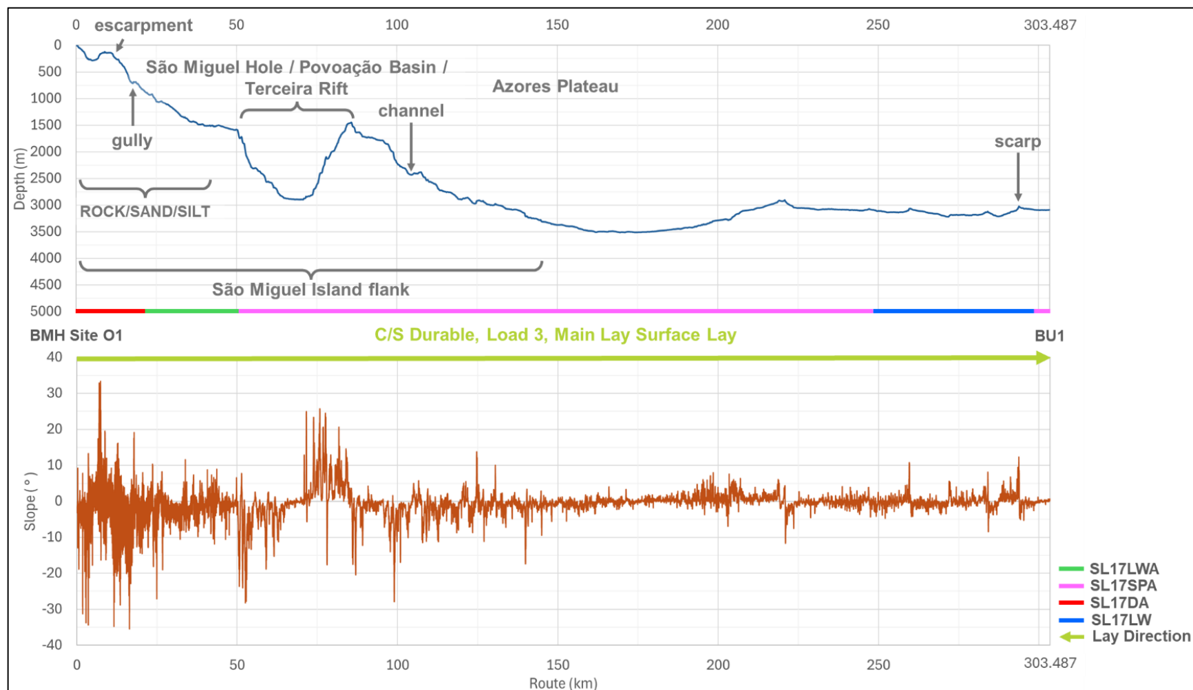
Figura 7.3 - Profundidade (batimetria) para instalação do cabo SOL e respetivas batimetrias para o segmento MARVEL S1.1 (Fonte: SubCom)
