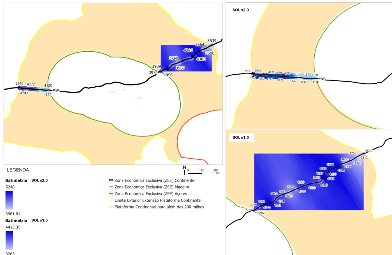
Figura 7.1 - Profundidade (batimetria) para instalação do cabo SOL e respetivas batimetrias nas zonas de atravessamento da PCE (Fonte: AECOM; Geoportal do Mar Português – DGRM, 2025)
