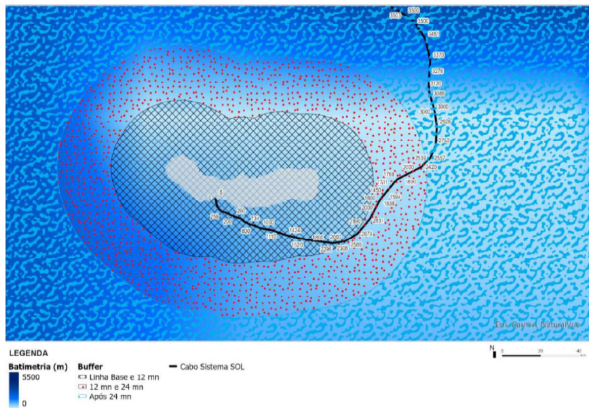
Figura 7.4 – Batimetria GEBCO - Ramal de ligação de São Miguel – Açores do cabo do Sistema SOL: BU1 – S1.1 (BMH) (Fonte: Geoportal do Mar Português)
